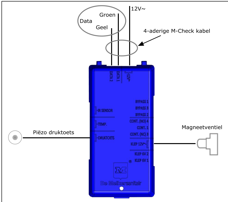
Afbeelding 4 Aansluitingen op de UCU (Toilet)
